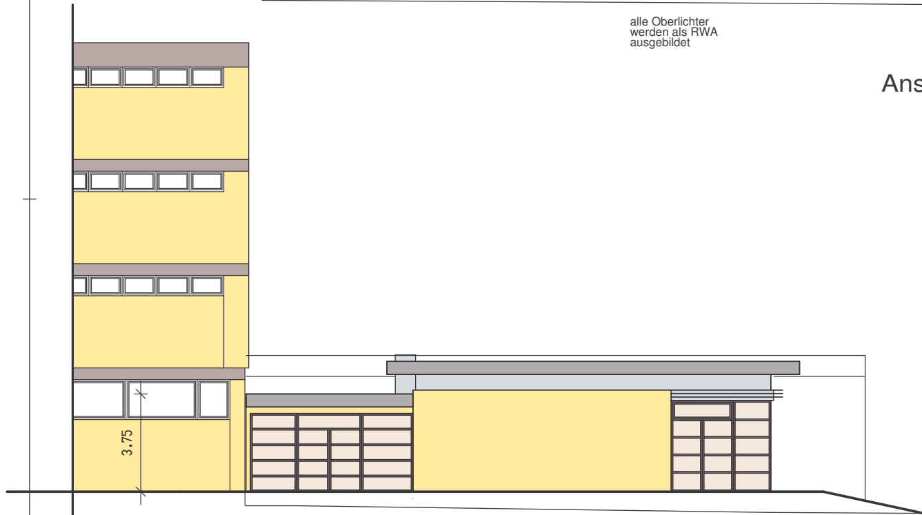
Ansicht Norden
