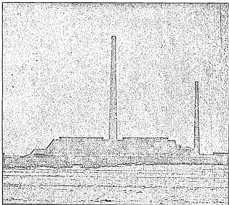
Schornstein 70 m hoch, 2,20 ob. l. Weite für Wicking'sche Portland-Cement- und Wasserkalkwerke Friedrichshorst bei Beckum, erbaut 1900.
